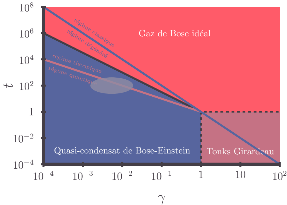
FIGURE II .4 – Diagramme des régimes principaux du gaz de Lieb–Liniger : gaz de Bose idéal, TG et qBEC , en fonction des paramètres adimensionnés \gamma et t . Les courbes noires, bleues et orange délimitent les cross-overs entre régimes. La zone grise correspond aux paramètres expérimentaux explorés pendant la thèse. Figure adaptée de [BDW11].
