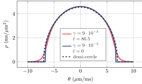
FIGURE II .3 – Distributions de rapidités pour différents paramètres de Lieb \gamma et différentes températures réduites t . Distribution dans le régime de faible interaction ( \gamma \ll 1 ) : le demi-cercle gris représente la distribution attendue pour \gamma \rightarrow 0 , tandis que le profil bleu correspond à \gamma petit mais non nul, montrant une discontinuité aux extrémités. La distribution en rouge illustre l'état excité au-delà de l'état fondamental, avec apparition d'ailes aux extrémités.
